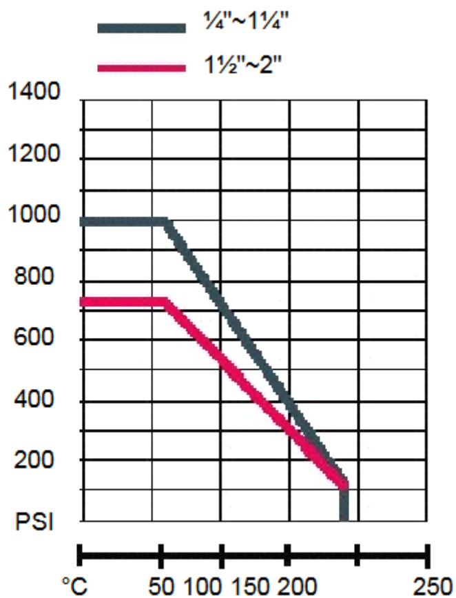
DIAGRAM ZÁVISLOSTI TEPLoty A TLAKU
